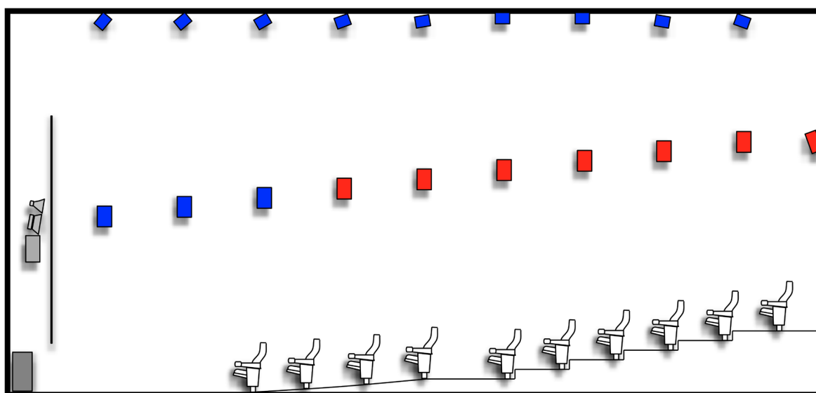
Figure 5.3 Emplacements de haut-parleurs plafond et latéraux recommandés
