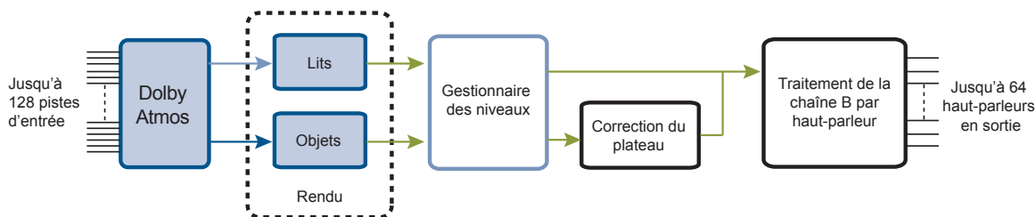
Figure 2.3 Diagramme du rendu Dolby Atmos
