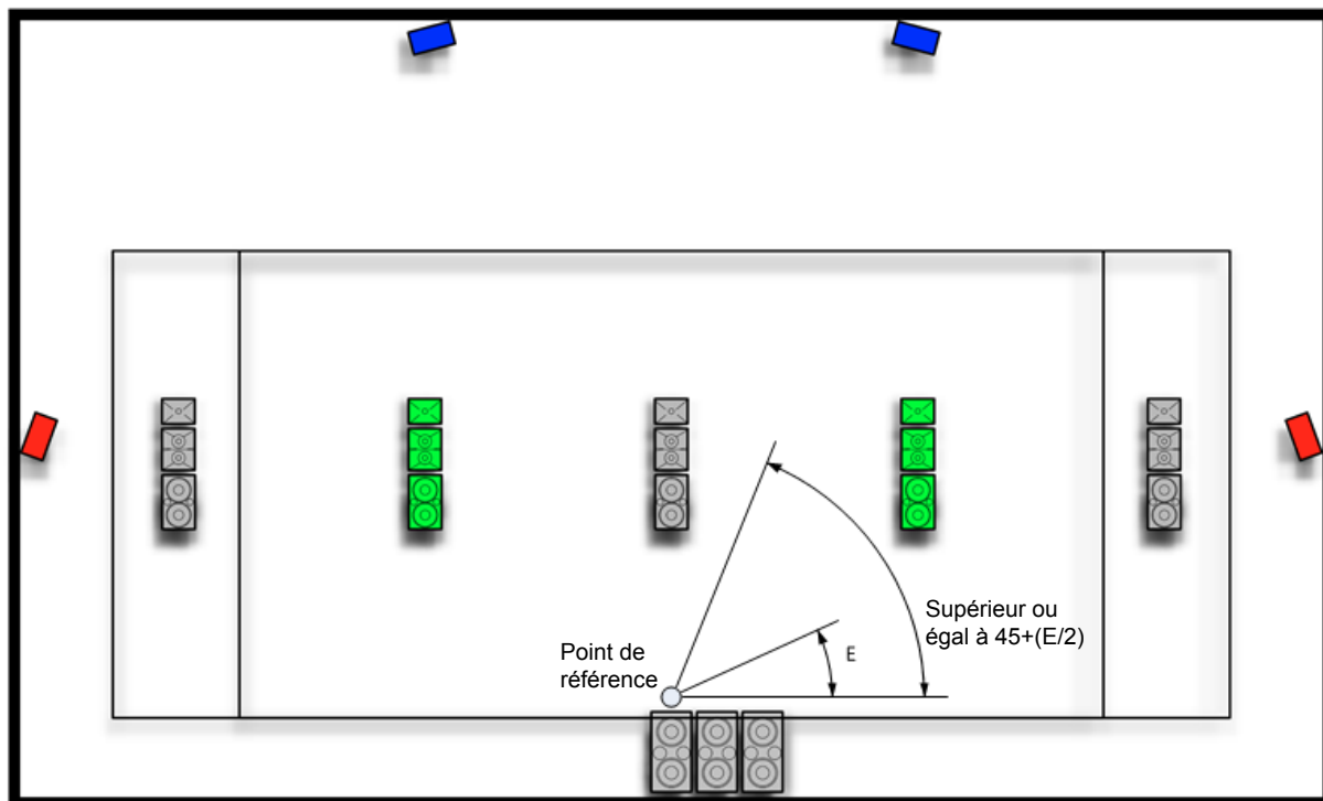
Figure 5.4 Exemple de position latérale des haut-parleurs plafond
