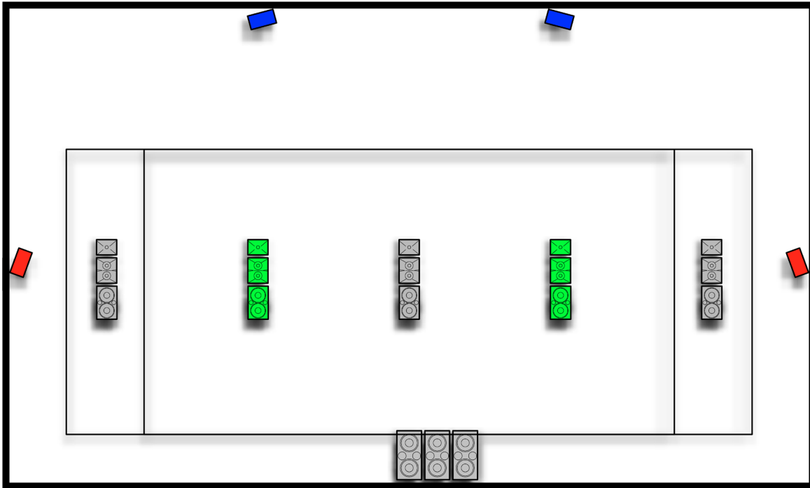
Figure 5.2 Emplacements de haut-parleurs recommandés (écran, surrounds latéraux et surrounds plafond)
